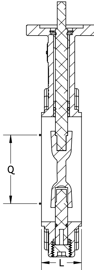
SECTION A-A
